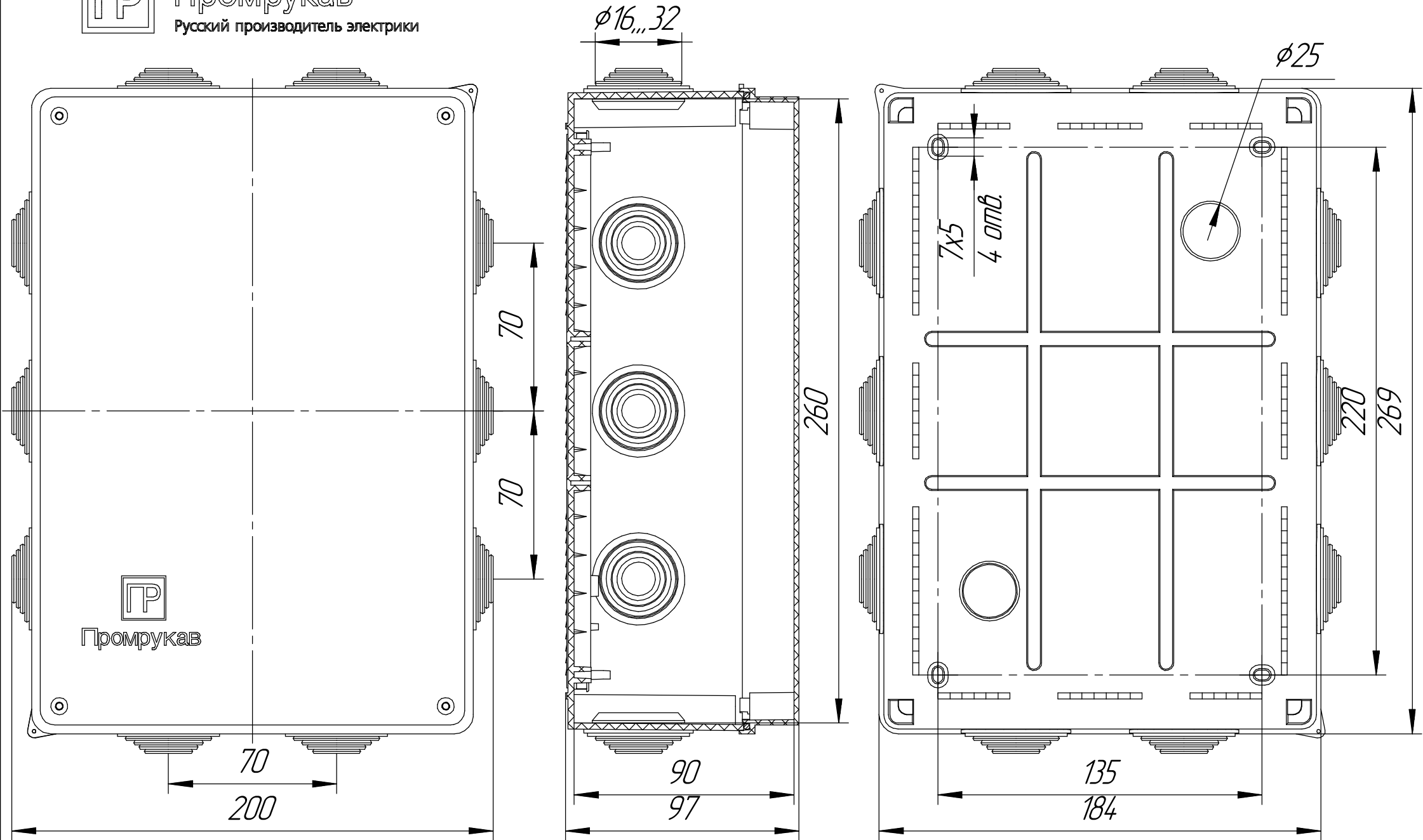
Коробка распределительная 40-0335 для о/п безгалогенная (HF) атмосферостойкая 260x175x90
