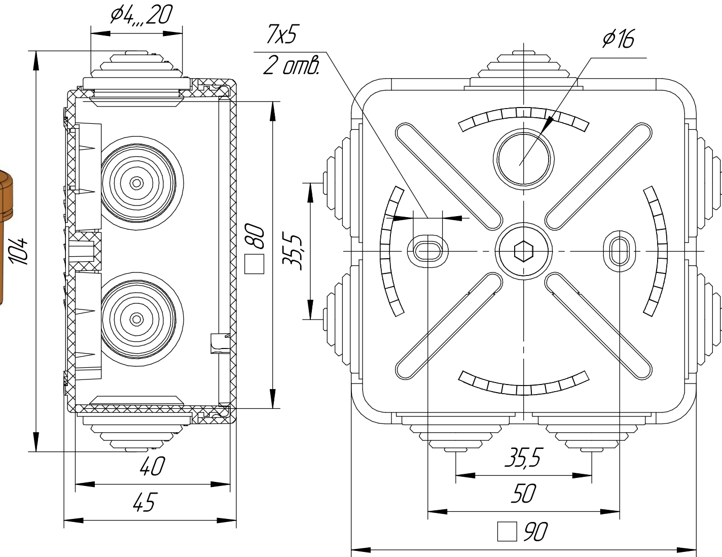
Коробка распределительная 40-0210-8001 для о/п безгалогенная (HF) б/к 80x80x40
