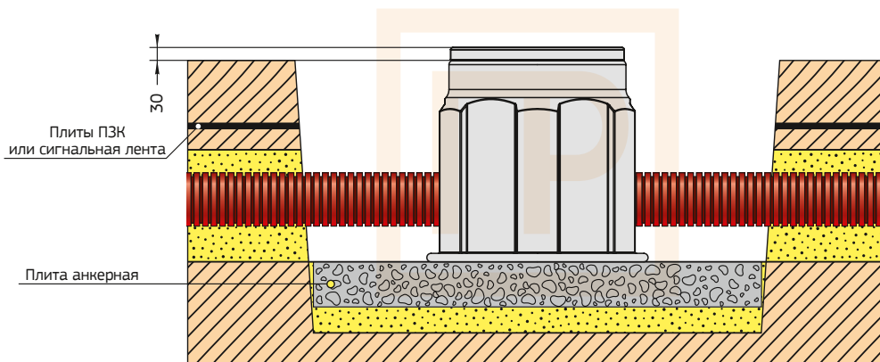
Рисунок №9. Установка вне проезжей части
