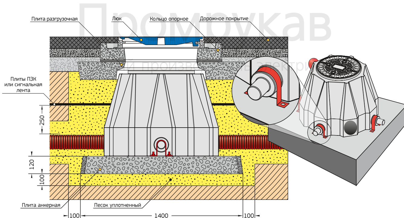
Рисунок №14. Установка под проезжую часть
