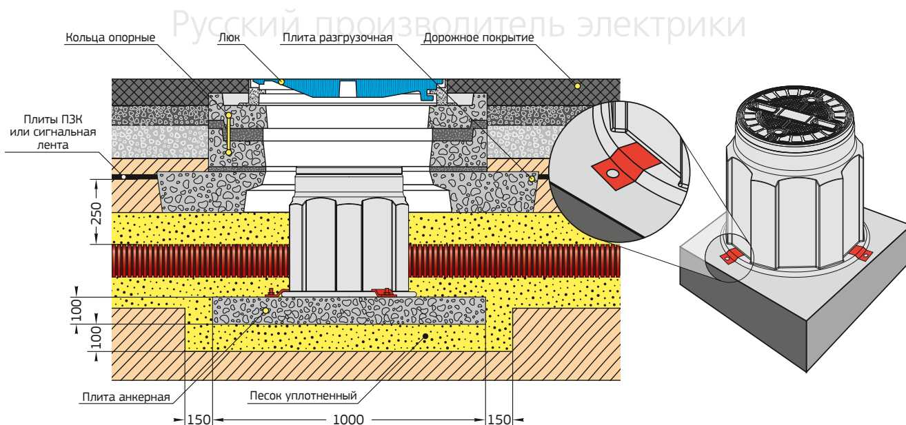
Рисунок №10. Установка под проезжую часть
